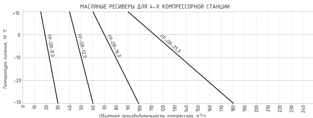
График 5. Подбор масляных ресиверов
