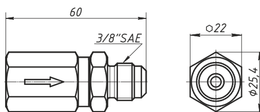
Дифференциальный обратный клапан. Differential check valve.
